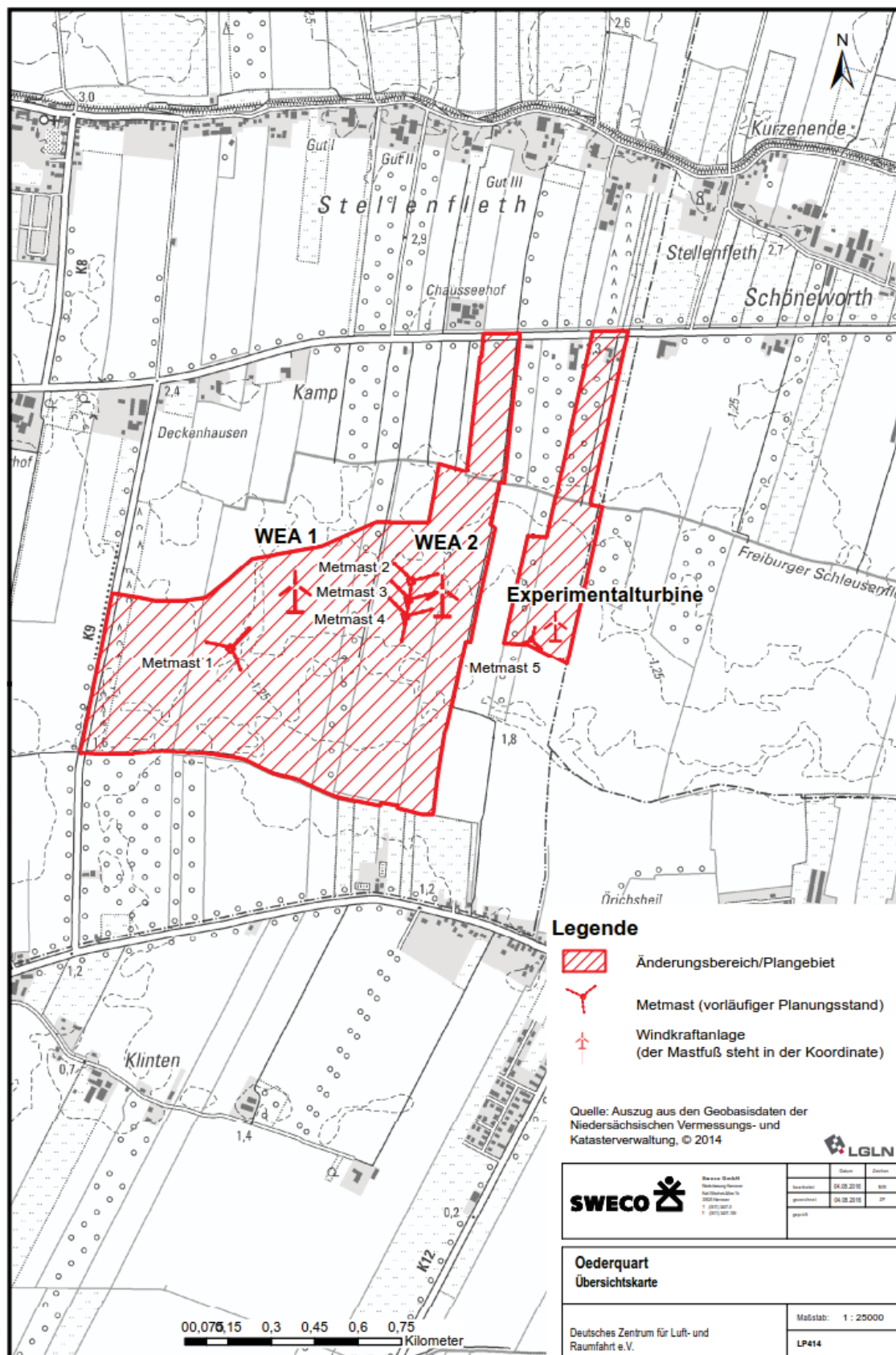
Abbildung 1: Übersichtskarte mit vorläufigem Aufstellungskonzept
